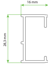
8 mm Tam Çerçeve Profili
