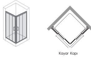
Köşe Kare / Dikdörtgen
