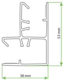
SOLVA - DESIGN PURE SAK YP Dönüş Profili
