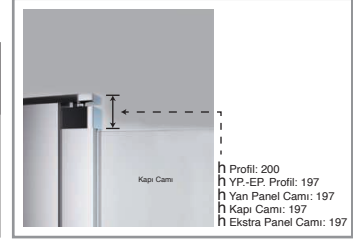
İçe Katlanır Kapı
