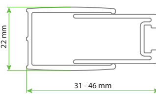
2. DESIGN PURE AK-SAK AKT - SOLVA SAK
